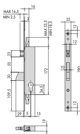
46250, 46252 E = 25 - 30 - 35
