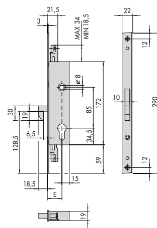
46265 E = 25 - 30 - 35
