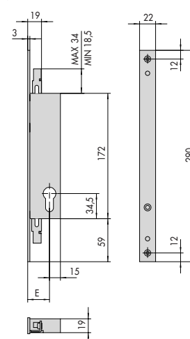
46270 E = 25 - 30 - 35
