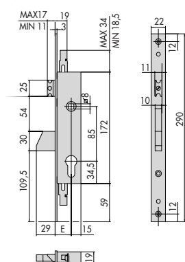
46225, 46227 E = 25 - 30 - 35
