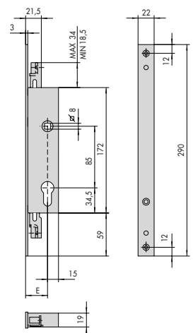
46275 E = 25 - 30 - 35
