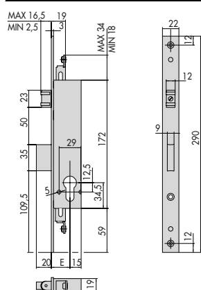
48250 E = 25 - 30 - 35
