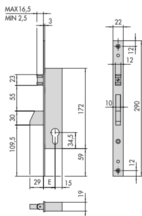
46230 E = 25 - 30 - 35
