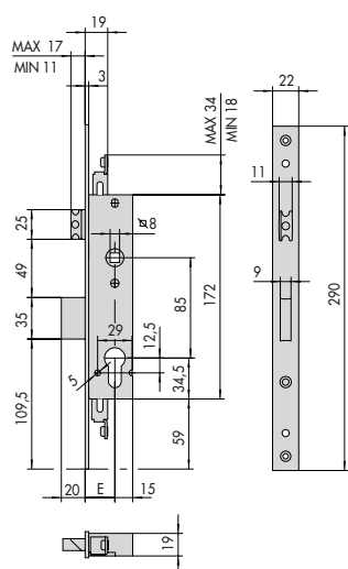
48225 E = 25 - 30 - 35
